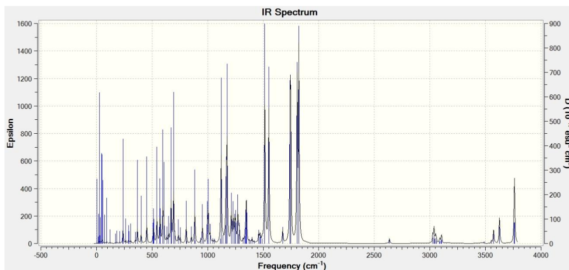
Рис.2 Теоретический ИК-спектр глутатиона
