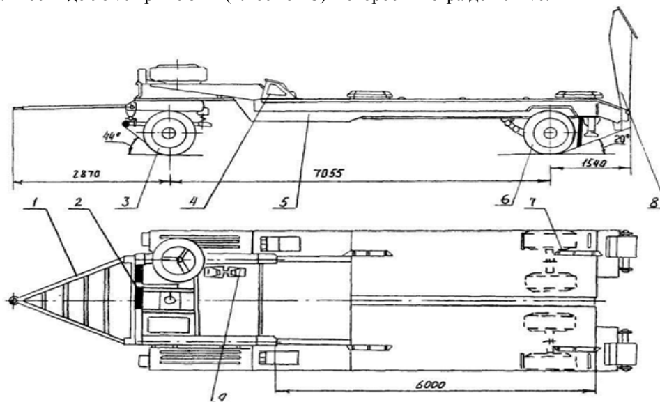
1 – дышло; 2 – направляющие ролики; 3 – подвеска передняя; 4 – упор; 5 – рама; 6 – колесо задняя подвеска; 7 – брус отбойный; 8 – трап; 9 – упор противооткатный
