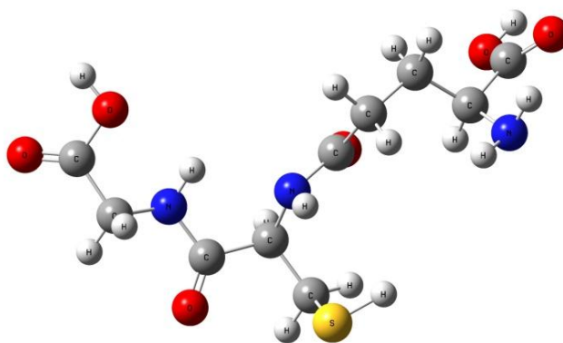
Рис. 1 Молекулярная модель глутатиона
