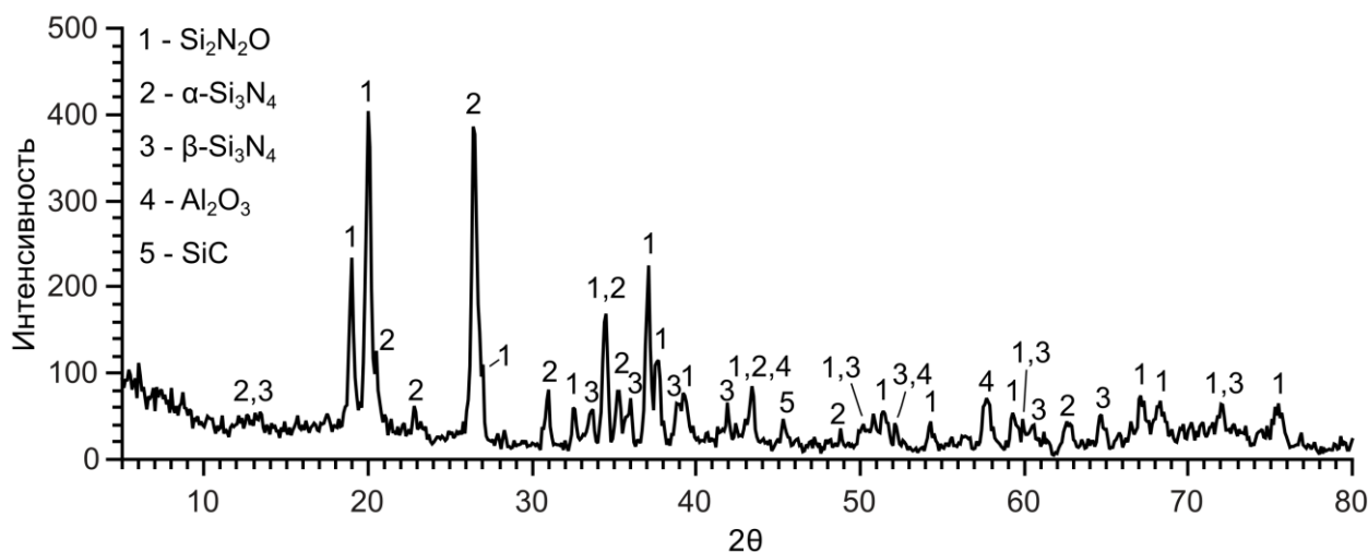
Рис. 2 – Дифрактограмма КМ-1 после спекания при T = 1320^\circ\text{C}
