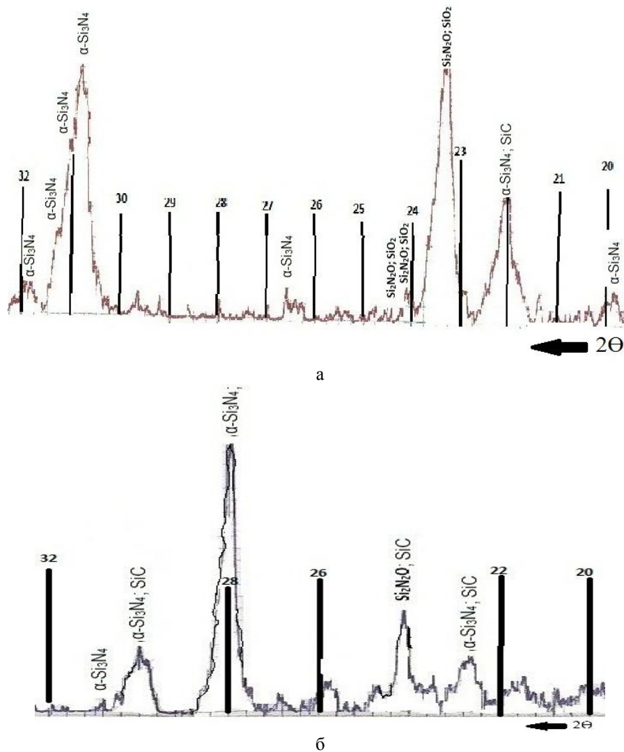
Рис. 1.а,б. Дифрактограмма керамокомпозиционного материала КМ-1 а- до воздействия агрессивной среды; б- после воздействия агрессивной среды.
