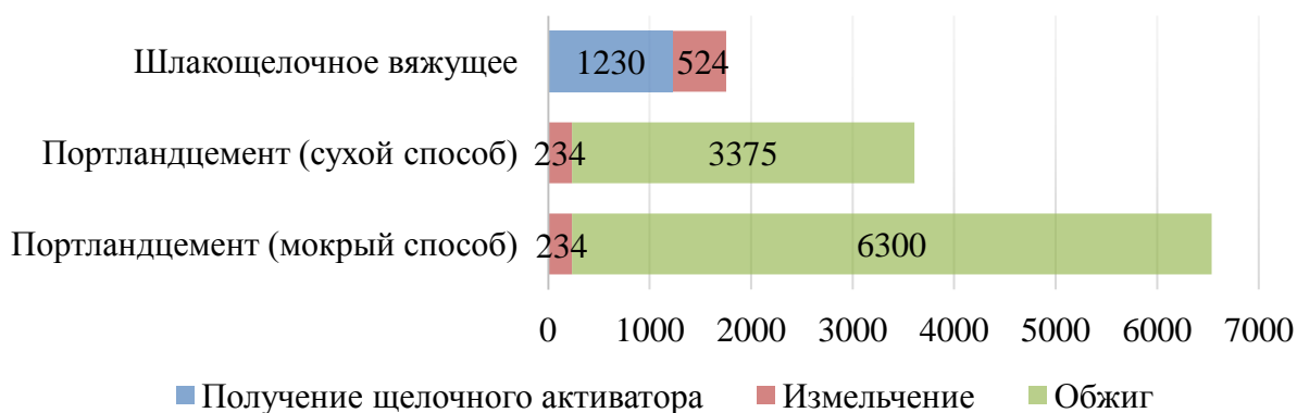
Рис. 1. Потребление энергии при производстве портландцемента и шлакощелочного вяжущего, МДж/т
