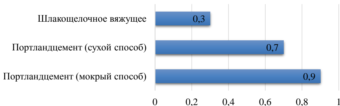
Рис. 2. Выбросы углекислого газа в атмосферу при производстве портландцемента и шлакощелочного вяжущего, т/т
