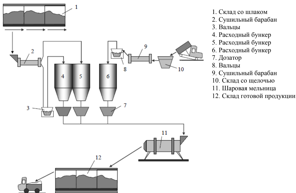
Рис. 3. Технологическая схема производства шлакощелочного вяжущего
