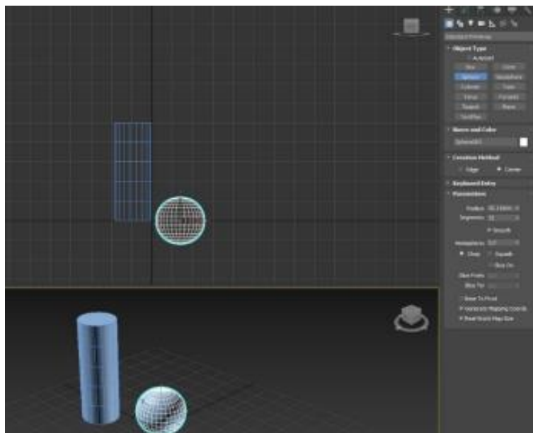
Рисунок 2. Создание примитивов
