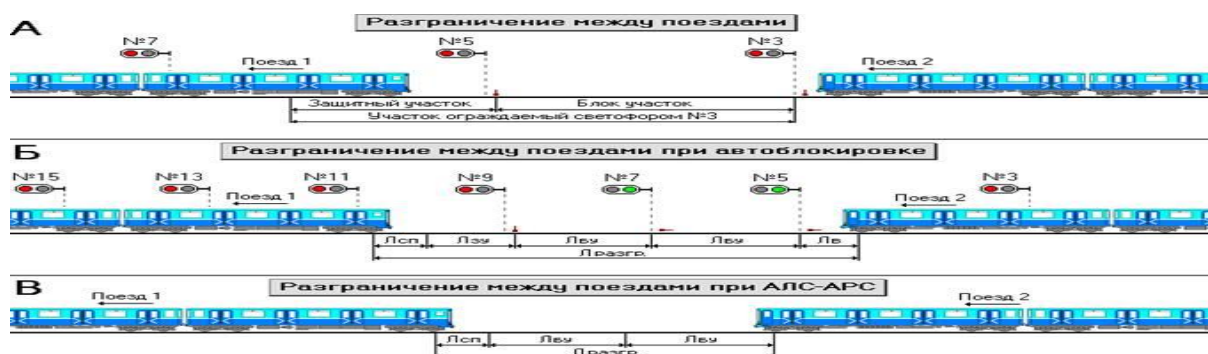
Рисунок 4. Система автоматического регулирования скорости (АРС)
