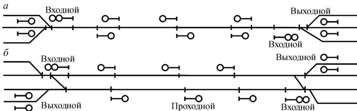
Рисунок 3. Система автоматической блокировки (САБ).
