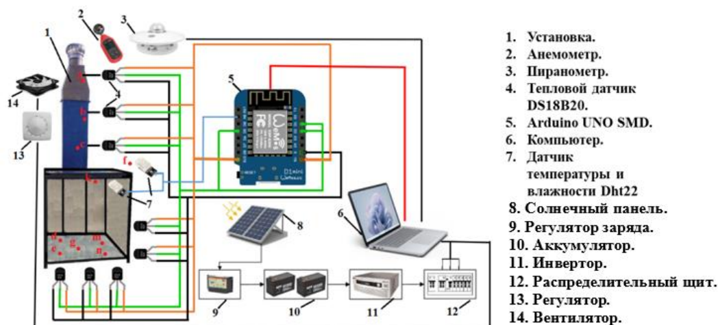
Рис. 1. Принципиальные схемы солнечной установки для опреснения воды.
