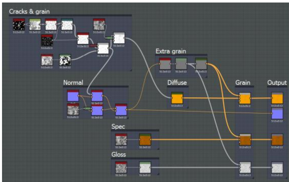
Рисунок 3. Граф
