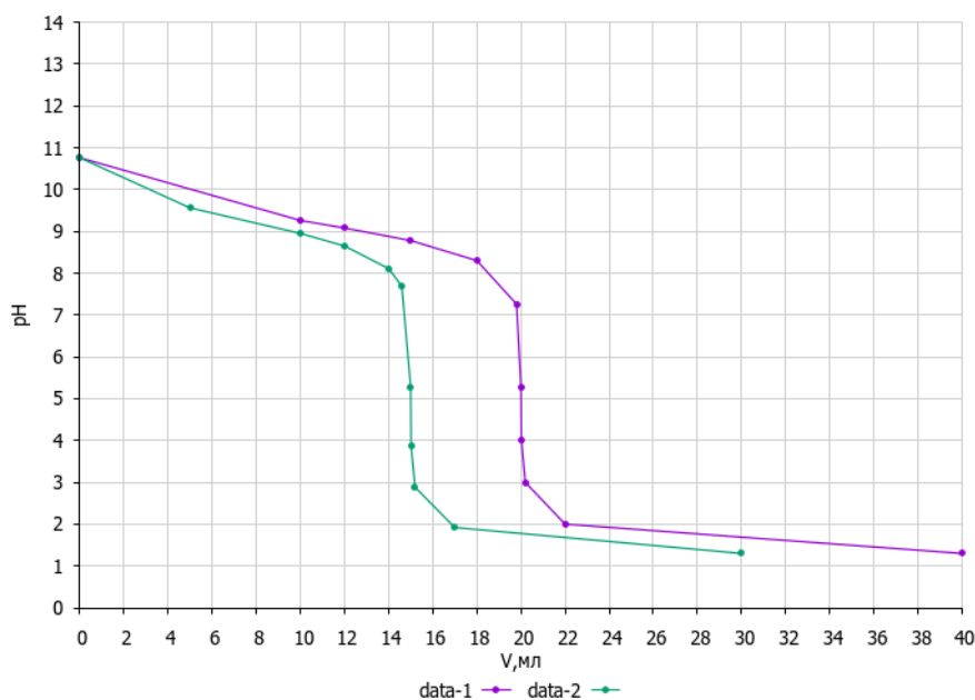
Рис.1 –Теоретические кривые титрования 0,1 М раствора гидроксида аммония 0,1 М раствором соляной кислоты по различным исходным объемам.
