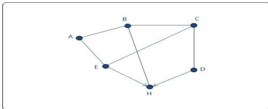
Рисунок 1. Граф
