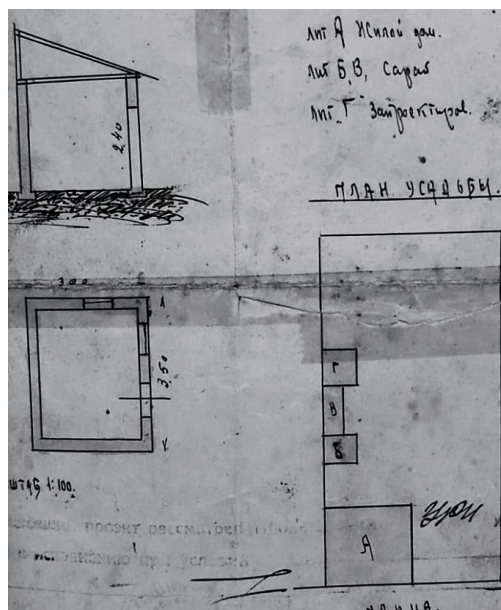
Рис. 5. Проект на постройку саманного сарая-кухни (1934 г.)
