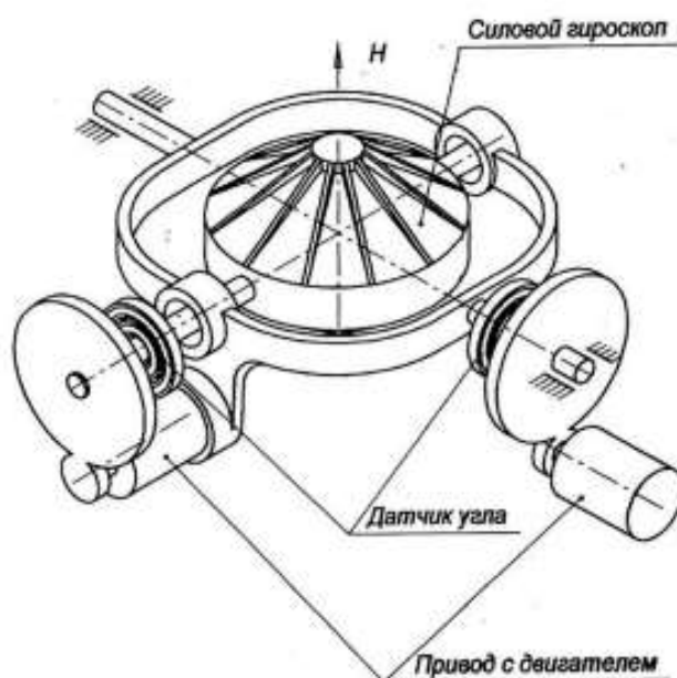
Рис. 6. Кинематическая схема трехстепенного силового гироскопа
