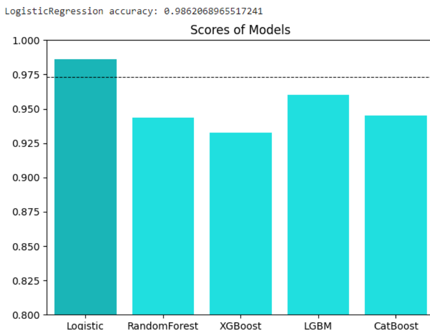
Рис. 3 – Оценка моделей
