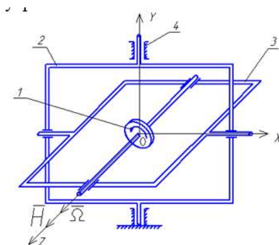
1 – Ротор; 2 – наружная рамка; 3 – внутренняя рамка; 4 – корпус прибора Рис. 1. Трехстепенной гироскоп
