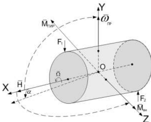
Рис. 2. Ротор гироскопа без рам карданова подвеса
