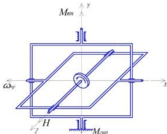
Рис. 4. Создание гирскопического момента у трехстепенного гироскопа
