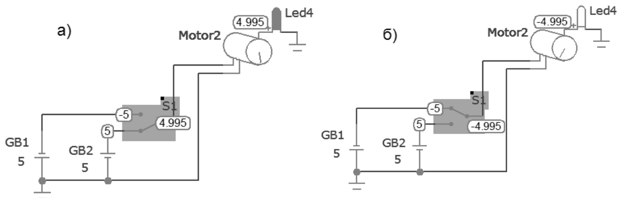
Рисунок 2 – Схемотехническая модель – двигатель постоянного тока и его реверсирование с индикацией.
