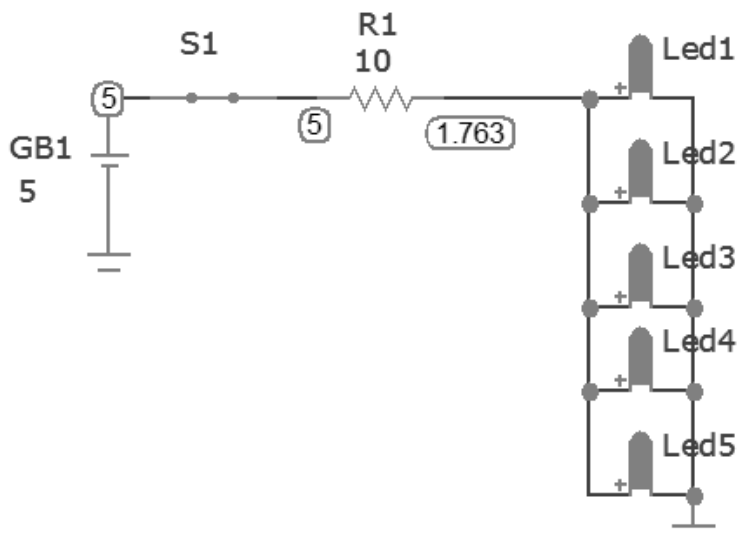
Рисунок 1 – Схемная реализация светодиодный фонарик.
