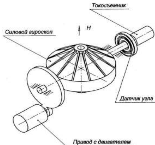
Рис. 5. Кинематическая схема двухстепенного силового гироскопа
