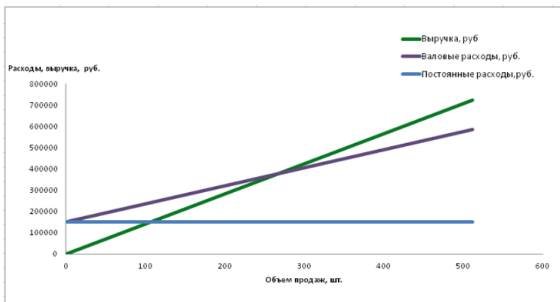
Рисунок 1 - График безубыточности
